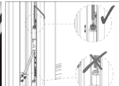
Höheneinstellung Schwerlastmodul Inside
